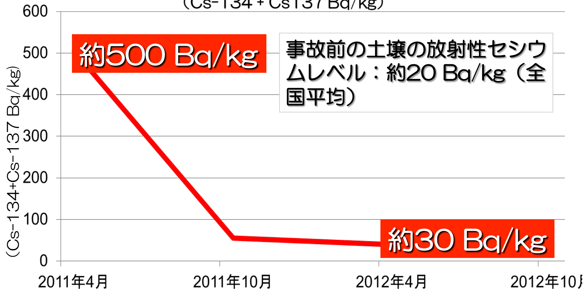
土壌（0-20cm）放射性セシウムレベル (Cs-134 + Cs-137 Bq/kg)
